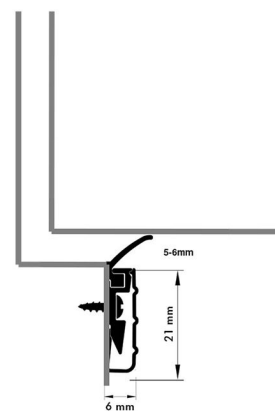
SA Holder with 097 Insert
