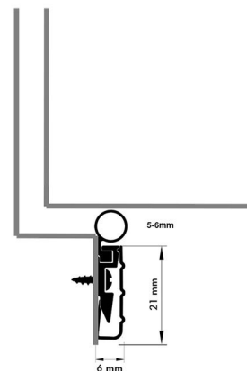
SA Holder with 089 Insert
